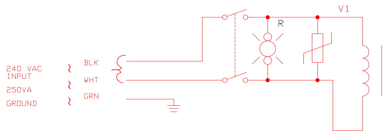
WIRING SCHEMATIC
